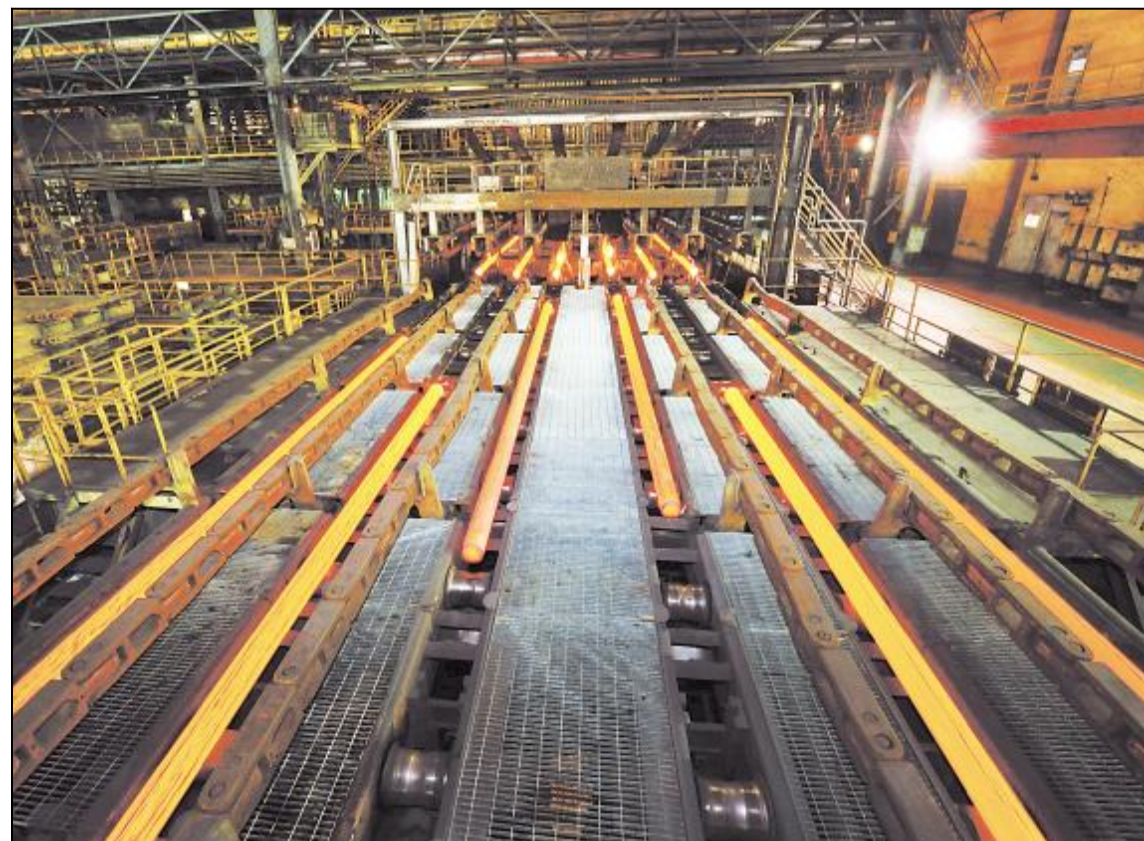
宝新钢加坡钢管事业部面对产销两旺、货源紧张的局面,年初从科学计划开工提升、操作改进和设备保障四个方面入手,将电炉“挑战”二百万吨吨位长坯列为年度重点工作。经过反复探索和磨合,五月份计划完成率提升百分之一百零三。图为连铸圆方坯浇铸生产线。记者 张勇 通讯员 彭玉洁 摄影报道
