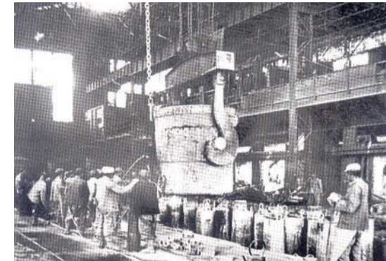
▲1952年9月，太钢冶炼出新中国第一炉不锈钢，并制成宝塔向党中央和毛主席报喜。
